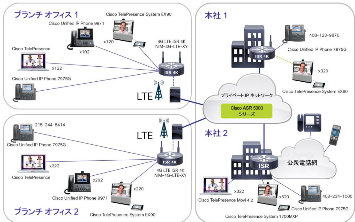
図 2. WAN のリスク分散を実現する Cisco LTE Advanced WWAN NIM
