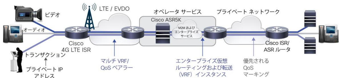
図 5. LTE Advanced マルチベアラー QoS
