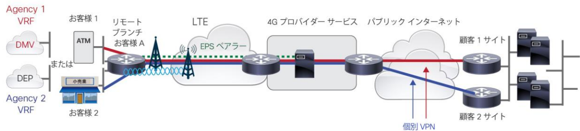
図 6. セルラーのマルチテナントまたはエージェンシー
