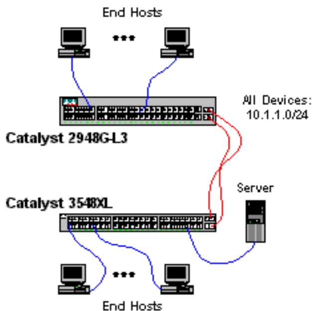
Figure 1 : Exemple 1 Diagramme de réseau
