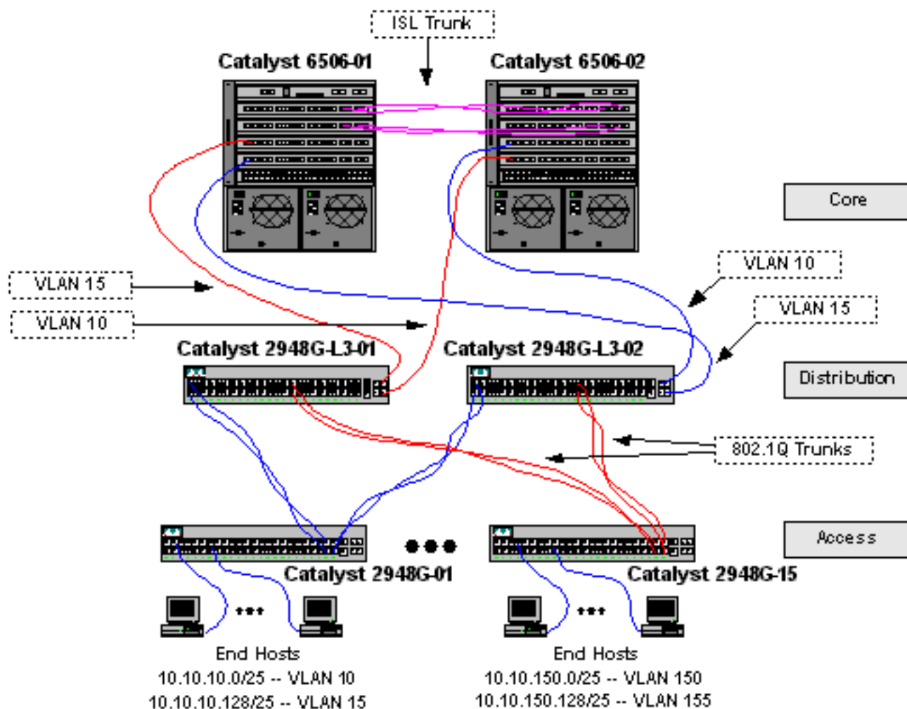
Figure 3 : Exemple 3 Diagramme de réseau
