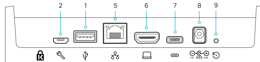
メインコネクタパネル (背面) (Desk)
